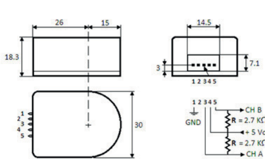
Encoder
