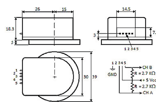
Encoder
